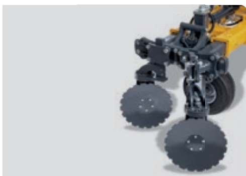
LAVORAZIONE A RICOLMARE: dischi ricolmatori indipendenti
