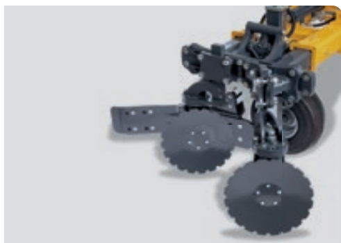
LAVORAZIONE A RICOLMARE (ALTERNATIVA): dischi ricolmatori indipendenti + lama paraterra
